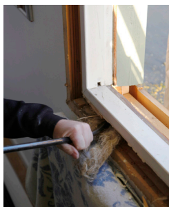
Gammal drevning petas fram och slängs.
